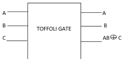
Fig.2: Toffoli gate.
