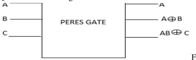
fig.1: Peres gate.
